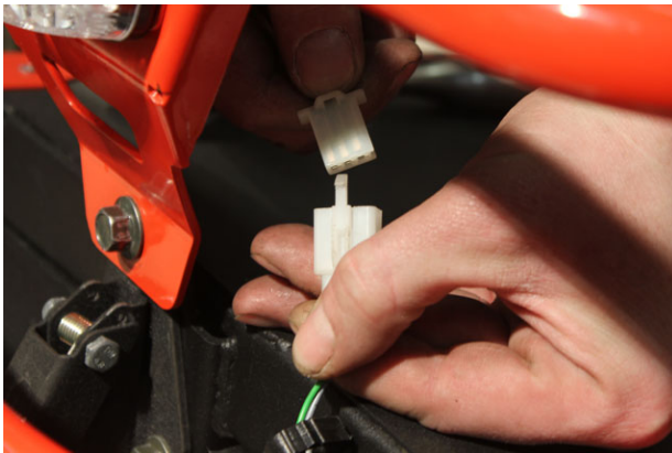
26. Разъединяем разъем заднего фонаря
