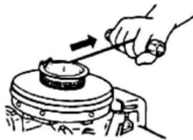
Фиксатор стартера
